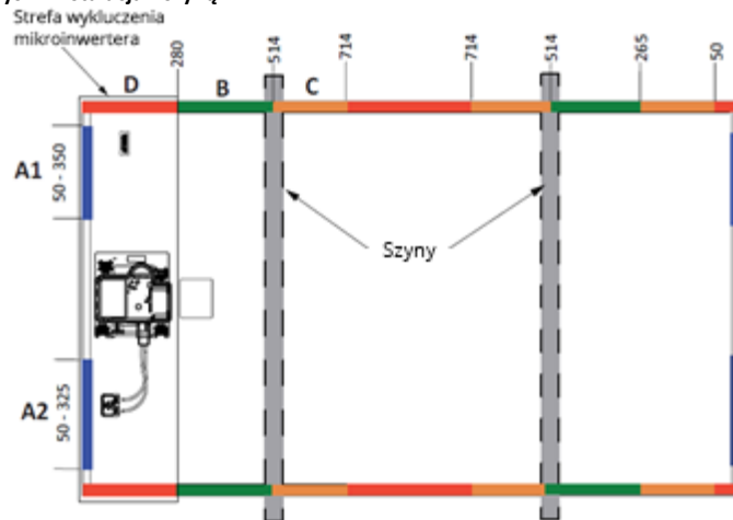
Rys. 2 Instalacja bez szyny
