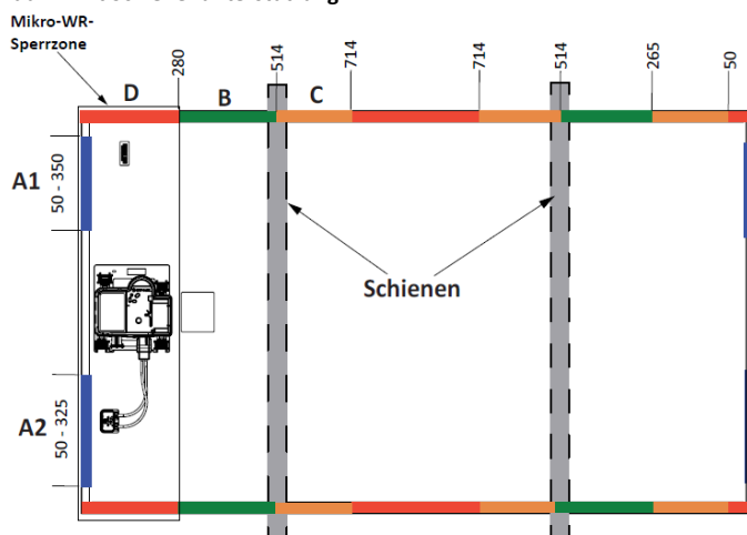
Abb. 1: Mit Schienenunterstützung
