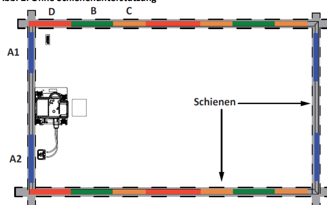
Abb. 2: Ohne Schienenunterstützung
