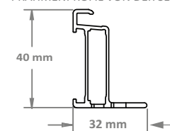
PROFILRAHMEN VON DER SEITE
