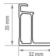
PROFIEL VAN ZIJFRAME
