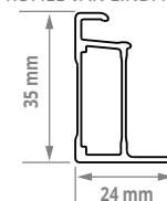
PROFIEL VAN EINDFRAME
