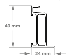
ENDE DES RAHMENPROFILS
