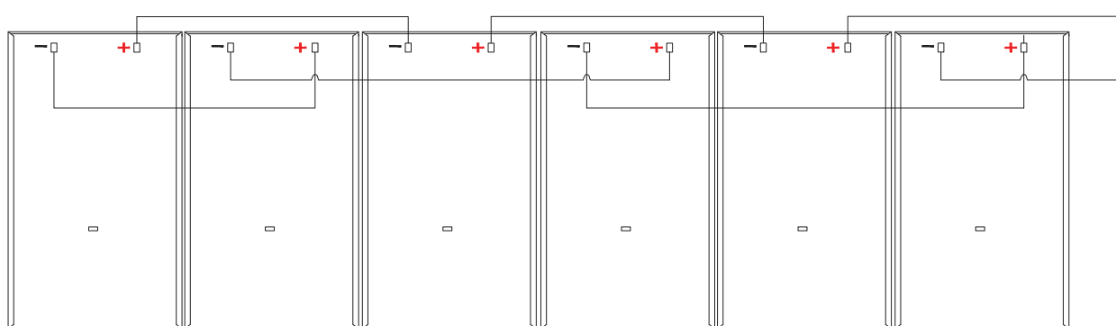
Leapfrog-Verkabelung (Hochformat)
